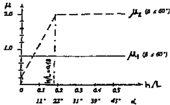
Fig. C.6.7 - Coefficienti di forma per differenti valori del rapporto altezza/lunghezza.
