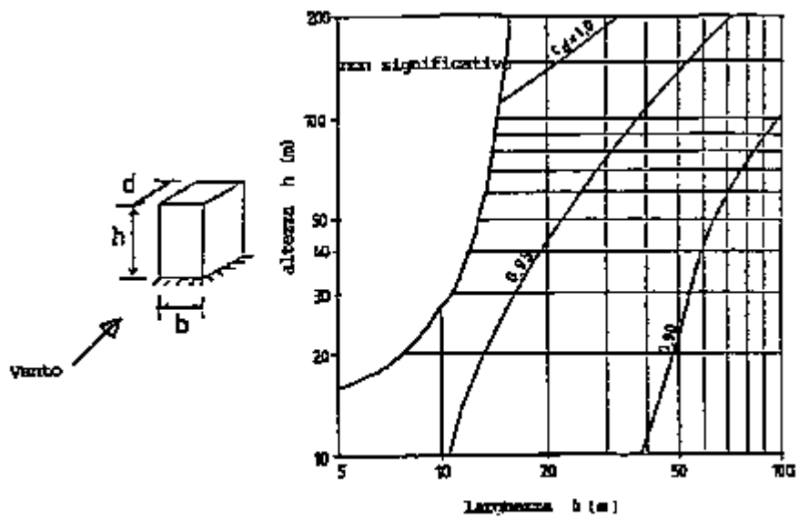
Fig. C.7.10 (a) - Edifici in ca. o in muratura.
